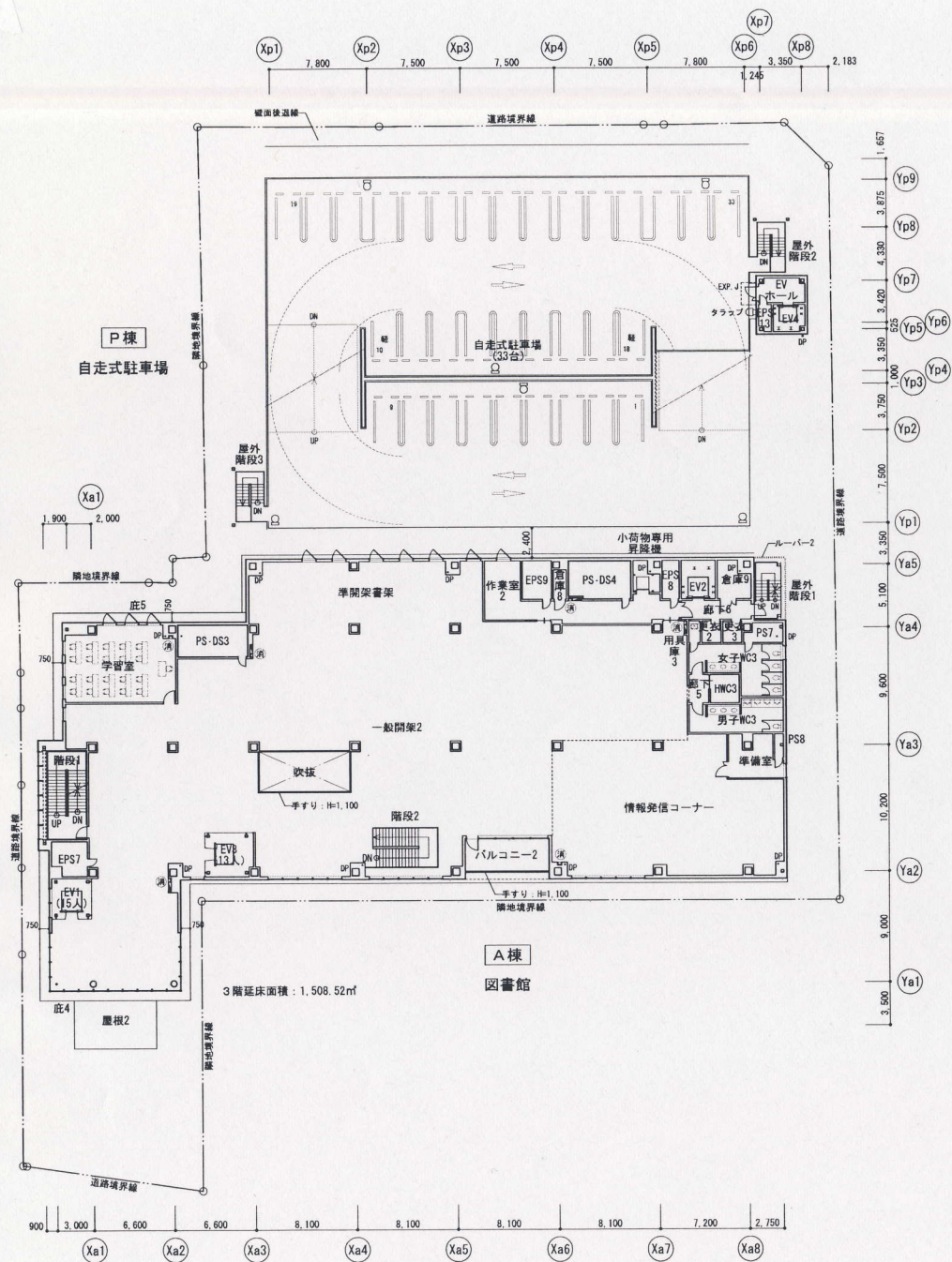
3階平面図 1/400
