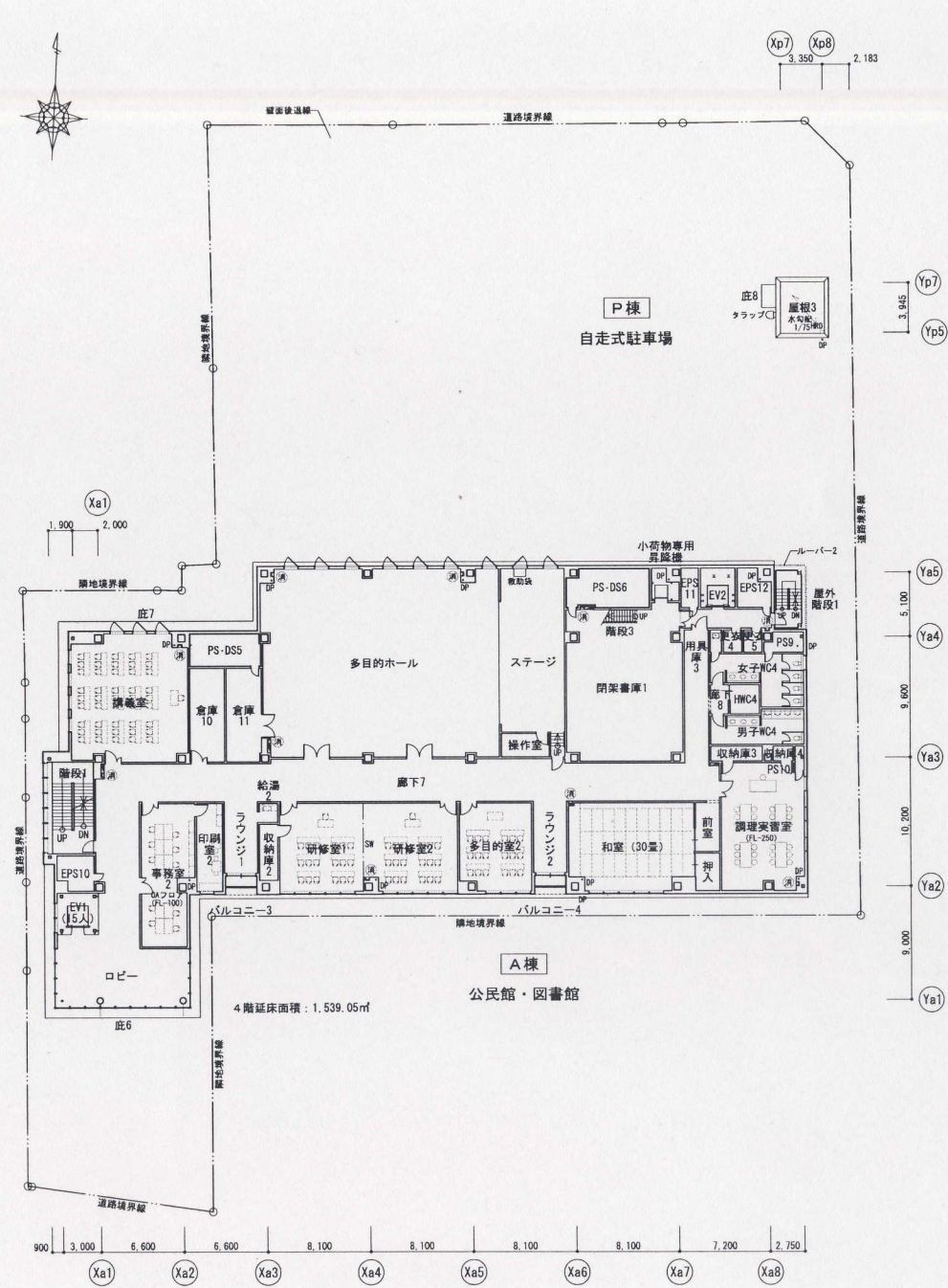
4階平面図 1/400
